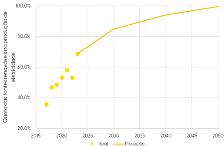
Figura 3.18 – Quotas das fontes renováveis na produção de eletricidade – dados reais até 2023 e projeção até 2050
